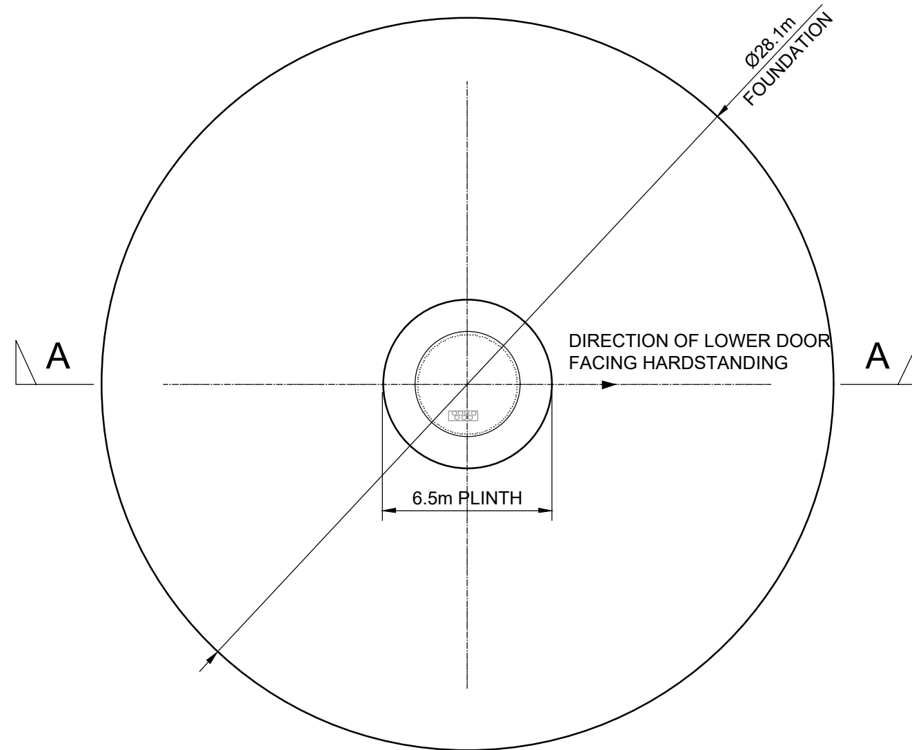
PLAN Scale: 1:200
